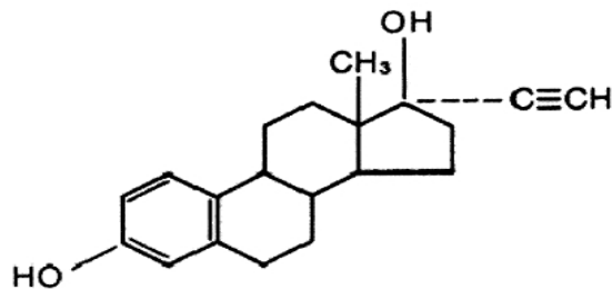
Ethinyl Estradiol C 20 H 24 O 2 MW: 296.4
