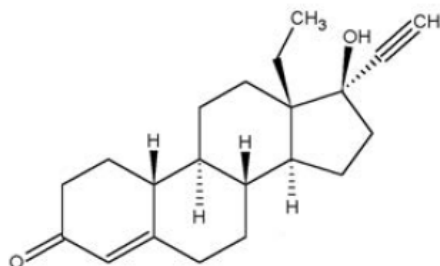
Levonorgestrel C 21 H 28 O 2 MW: 312.4
