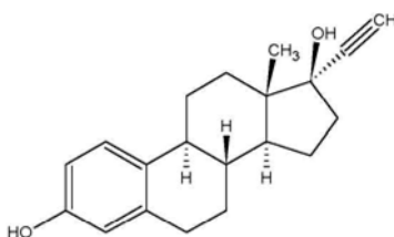
Ethinyl Estradiol
